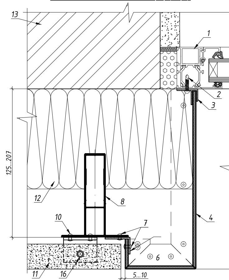
Горизонтальный разрез (3 а-3 а)
