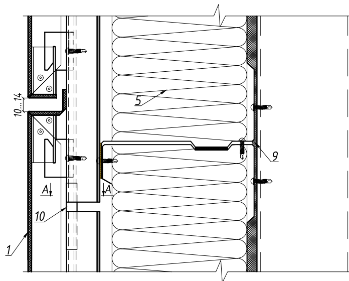
Стыковка стоек АК-1 по высоте
