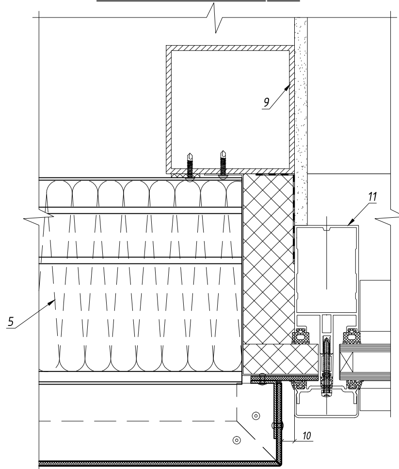
Горизонтальный разрез (6-6)
