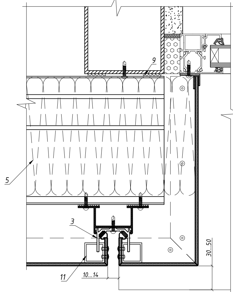
Горизонтальный разрез (3-3)
