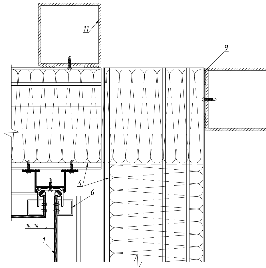
Внутренний угол (10-10)
