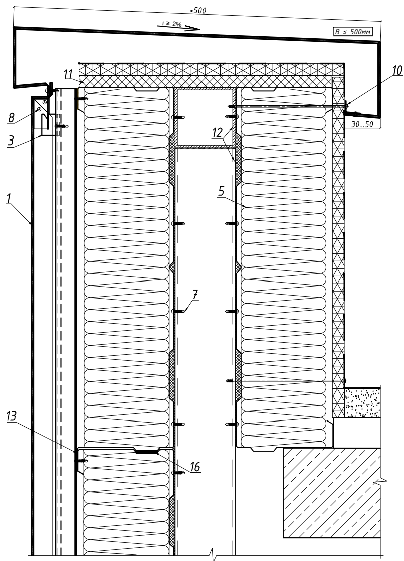
Вертикальный разрез (12 а - 12 а)
