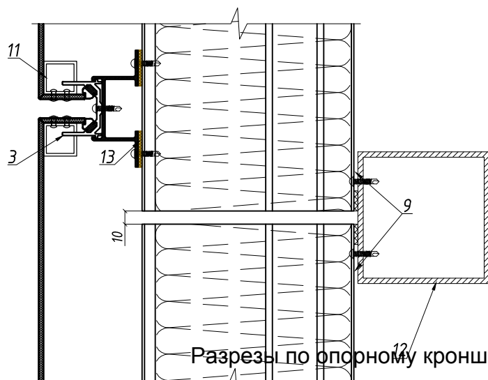
Горизонтальный разрез (2-2)
