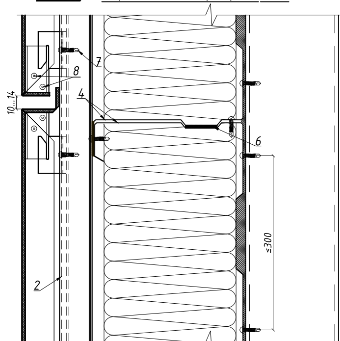
Горизонтальный разрез (2-2)
