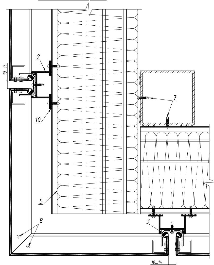
Внешний угол (9-9)
