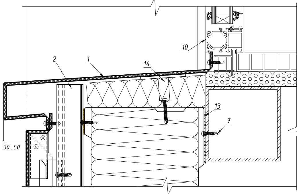
Вертикальный разрез (5-5)
