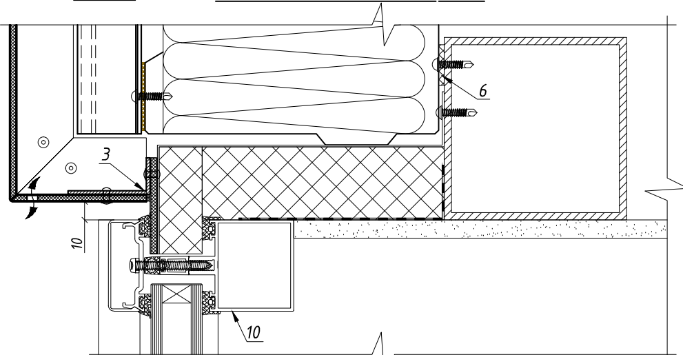
Вертикальный разрез (7-7)
