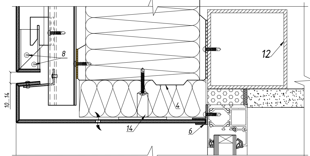
Вертикальный разрез (5-5)
