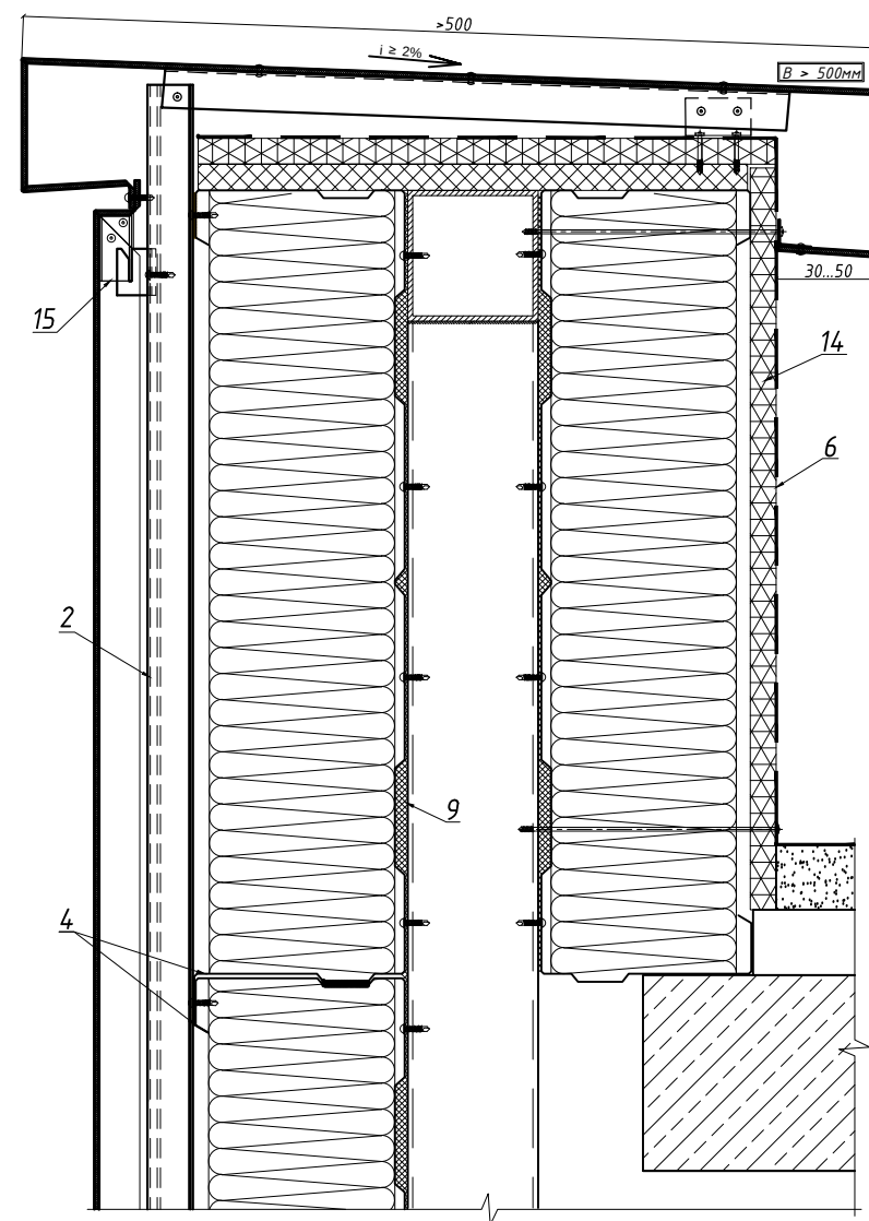
Вертикальный разрез (12 б - 12 б)
