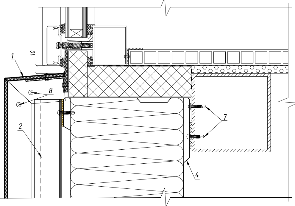
Вертикальный разрез (8-8)
